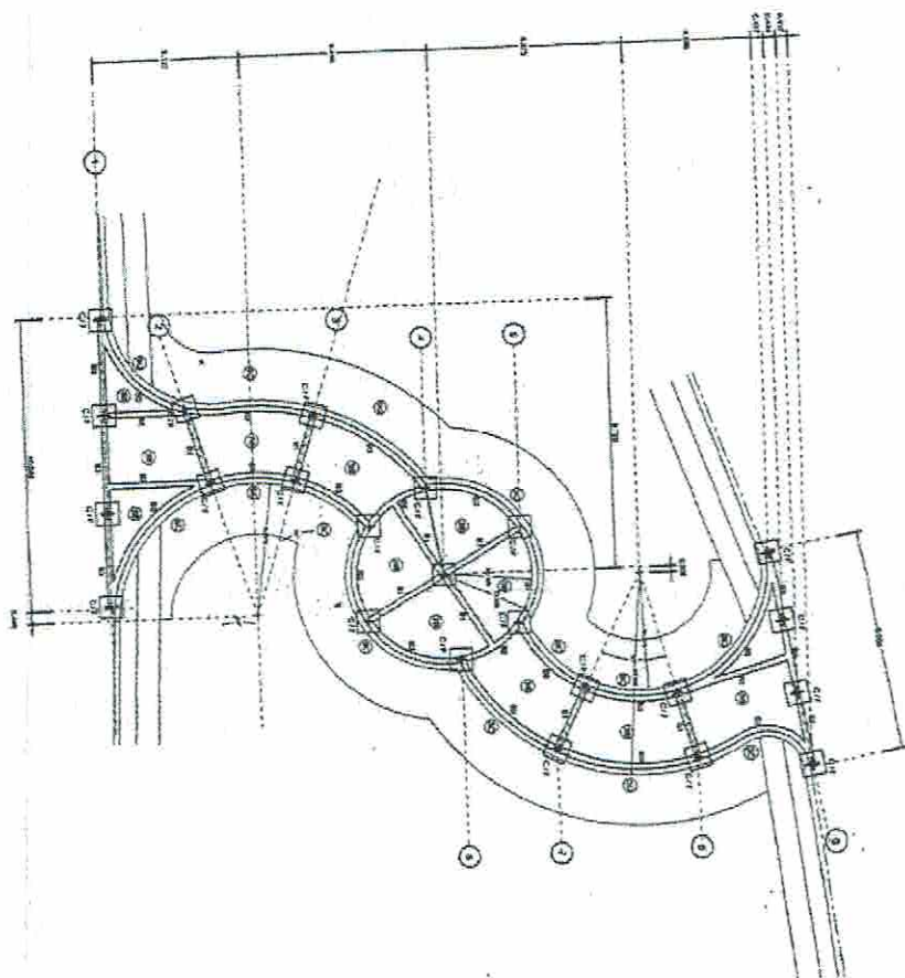
แบบแปลนอาคารหลัก (อาคารที่ ๑) ๑:๑๐๐
