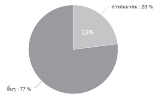
การปล่อย CO 2 เฉพาะภาคการใช้พลังงาน
