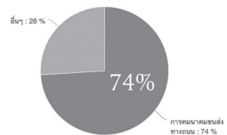
การปล่อย CO 2 เฉพาะด้านการคมนาคม
