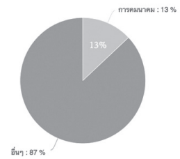
การปล่อย CO 2 ในระดับโลก
